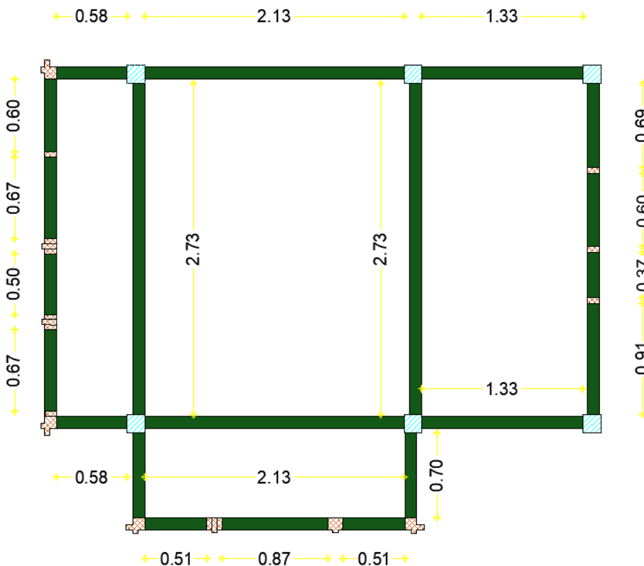
Εικόνα 5: Δοκάρια στο ύψος του ταβανιού του κτιρίου
