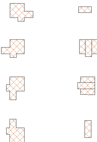
Εικόνα 6: Διαφορετικές διατομές ξύλινων υποστυλωμάτων τοιχοποιίας φυλακίου
