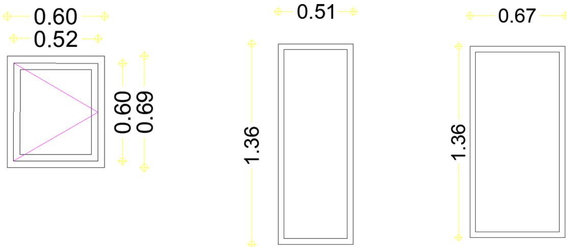
Εικόνα 8: Εξωτερικά παράθυρα φυλακίου με ανοιγόμενα και σταθερά τμήματα
