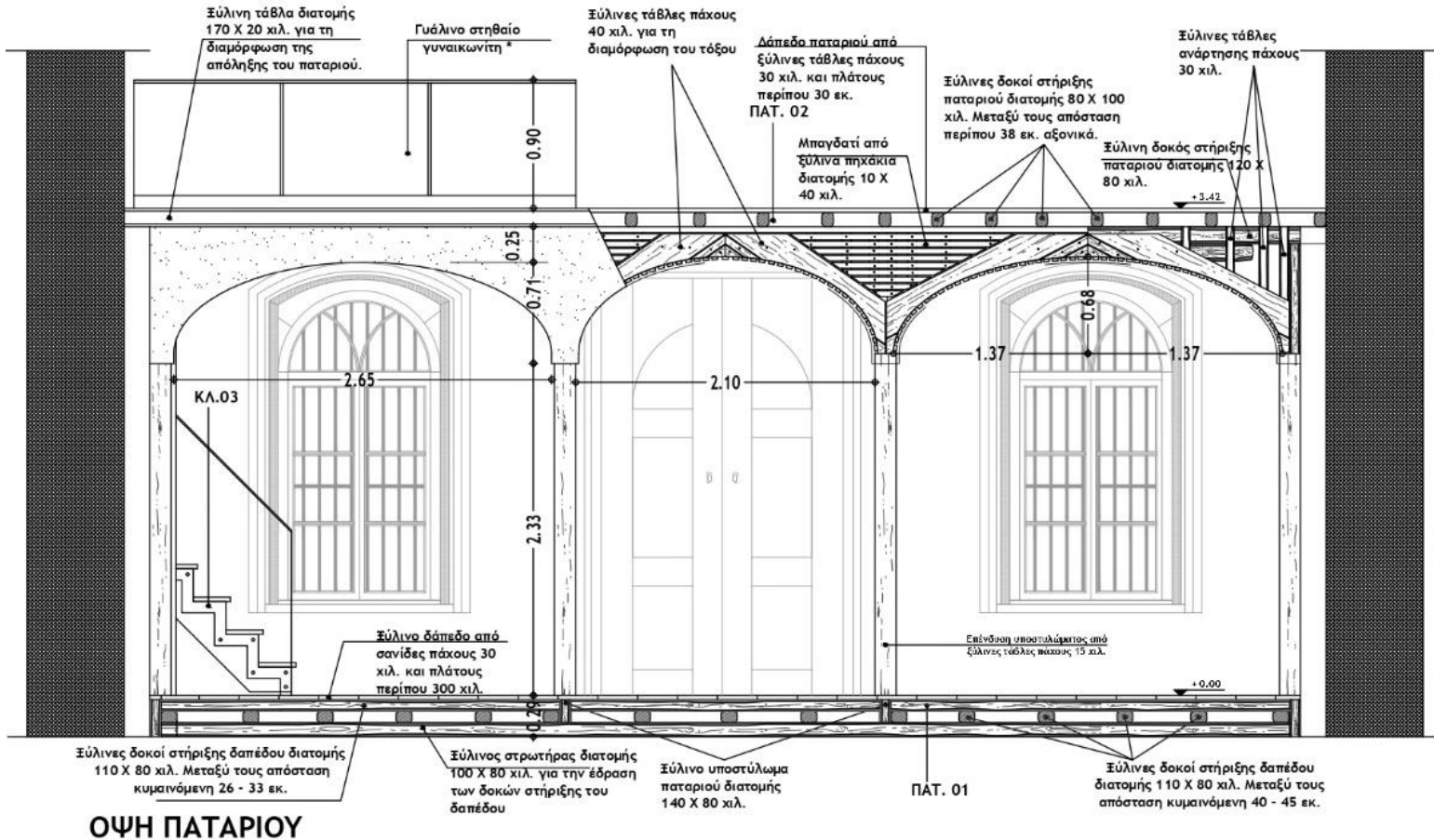
Σχέδιο 18 – Ώψη παταριού/ γυναικωνίτη
