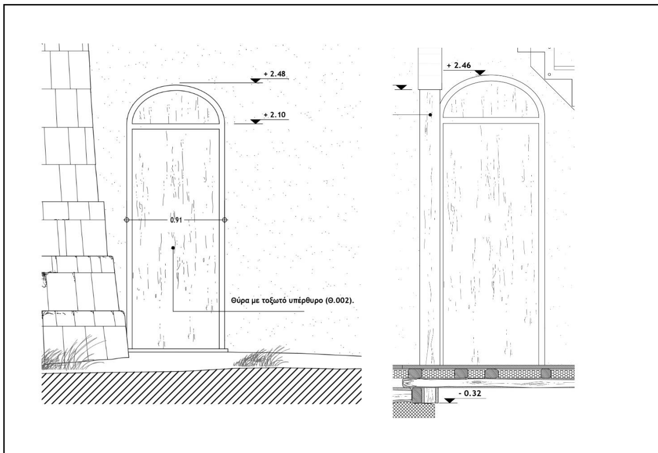
Σχέδιο 9 – Κούφωμα εισόδου (θ.002) στη βορειοδυτική πλευρά του κτιρίου (όψεις εξωτερικά και εσωτερικά)
