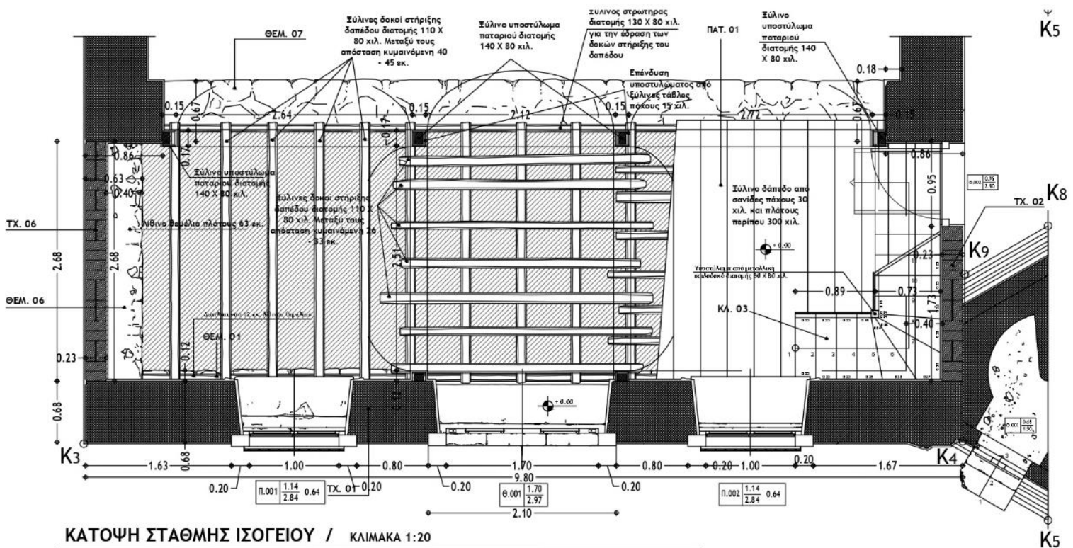
Σχέδιο 15 – Κάτοψη ισογείου στάθμη: 0.00μ (κάτω από το πατάρι/γυναικωνίτη)
