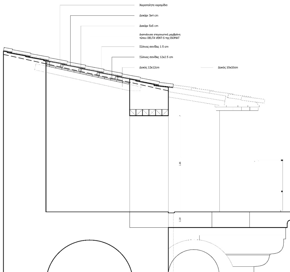
Λεπτομέρεια κατασκευής και επικάλυψης ξύλινης στέγης.
