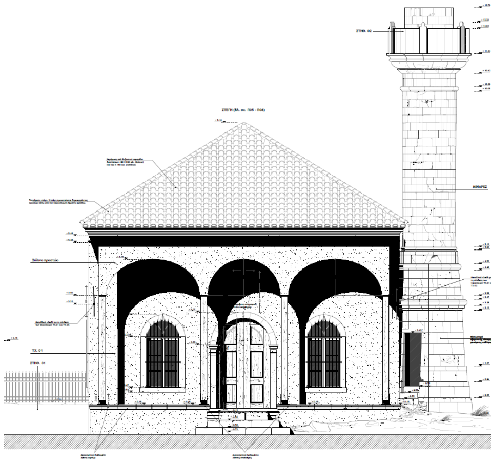
Σχ. 5-6 Ενδεικτική ανατολική και βόρεια όψη τεμένους
