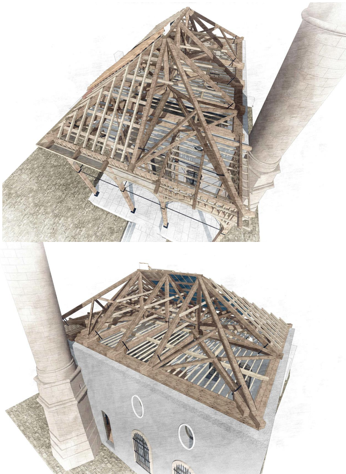
Εικ. 4-5. Τρισδιάστατες απεικονίσεις φέροντος οργανισμού στέγης
