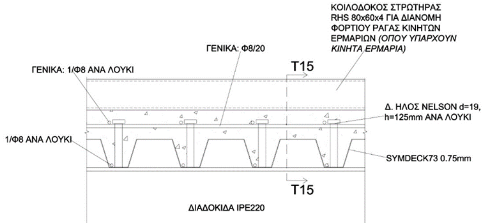
Εικόνα 11: Λεπτομέρεια σύμμικτης πλάκας οροφής ισογείου με λαμαρίνα SYMDECK73
