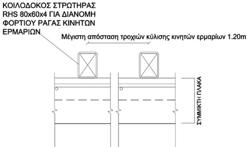
Εικόνα 12: Λεπτομέρεια στρωτήρα κοιλοδοκού στη σύμμικτη πλάκα σε σημεία τοποθέτησης κινητών ερμαρίων.
