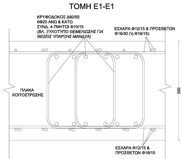
Εικόνα 5: Λεπτομέρεια όπλισης πλάκας θεμελίωσης.
