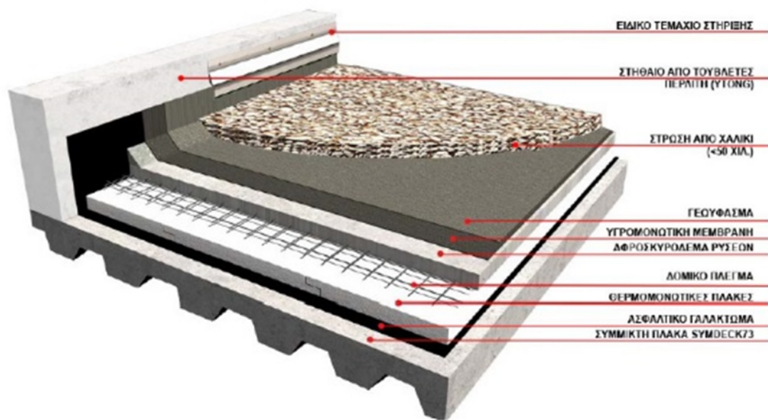
Εικόνα 13: Λεπτομέρεια διάστρωσης υλικών επικάλυψης δώματος
