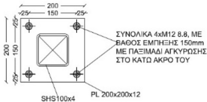
Εικόνα 10: Λεπτομέρεια έδρασης υποστυλώματος και αγκύρωσής του στις εδαφόπλακες του κλιμακοστασίου.
