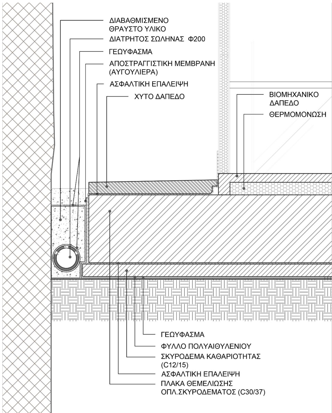
Εικόνα 4: Λεπτομέρεια θεμελίωσης
