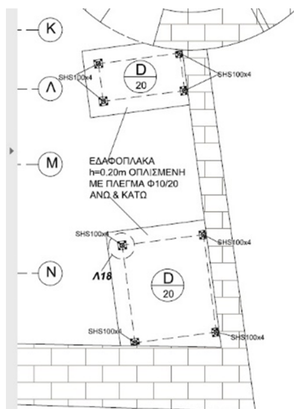
Εικόνα 9: Εδαφόπλακες πάχους 0,20m στην ανατολική πλευρά του κτιρίου για το εξωτερικό κλιμακοστάσιο.
