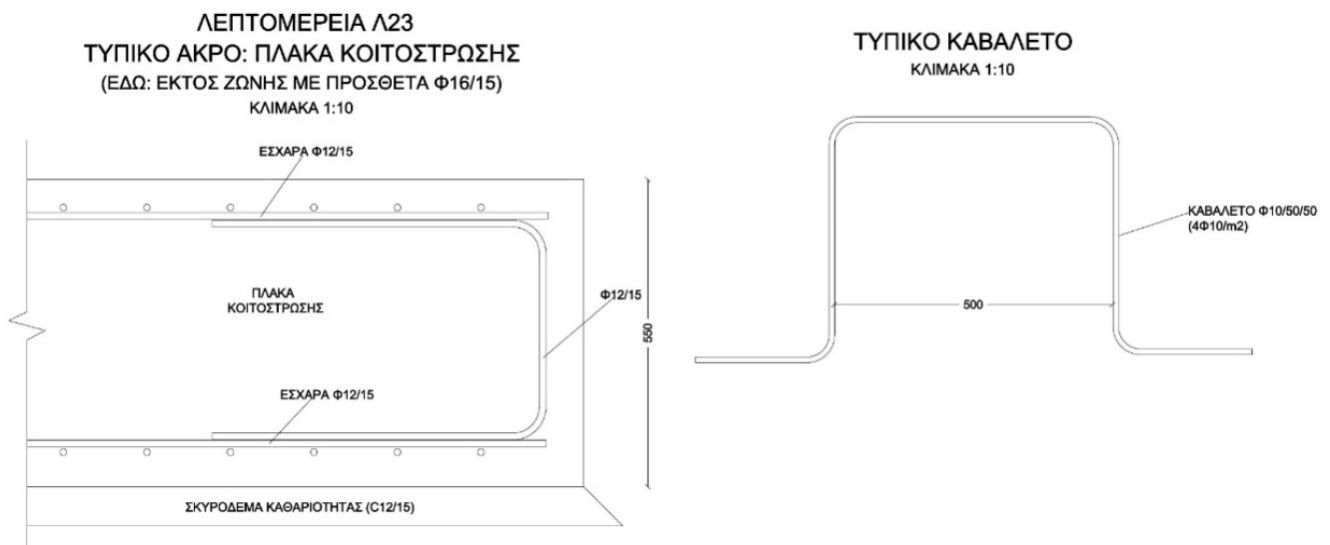
Εικόνα 5: Λεπτομέρεια όπλισης πλάκας θεμελίωσης.
