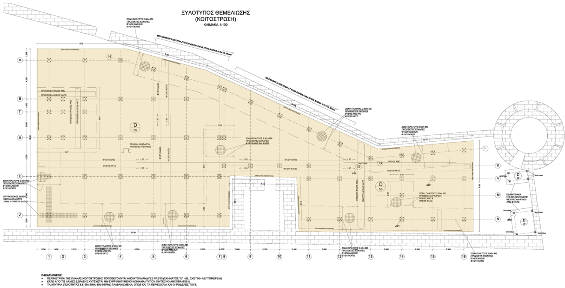
Εικόνα 3: Κάτοψη θεμελίωσης. Σημειώνεται με χρώμα η επιφάνεια που θα σκυροδετηθεί.
