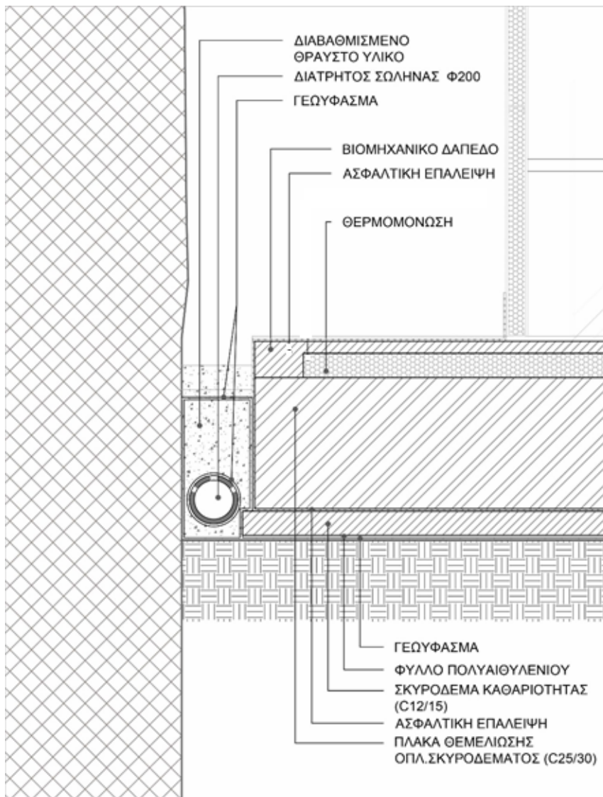
Εικόνα 3: Λεπτομέρεια θεμελίωσης.
