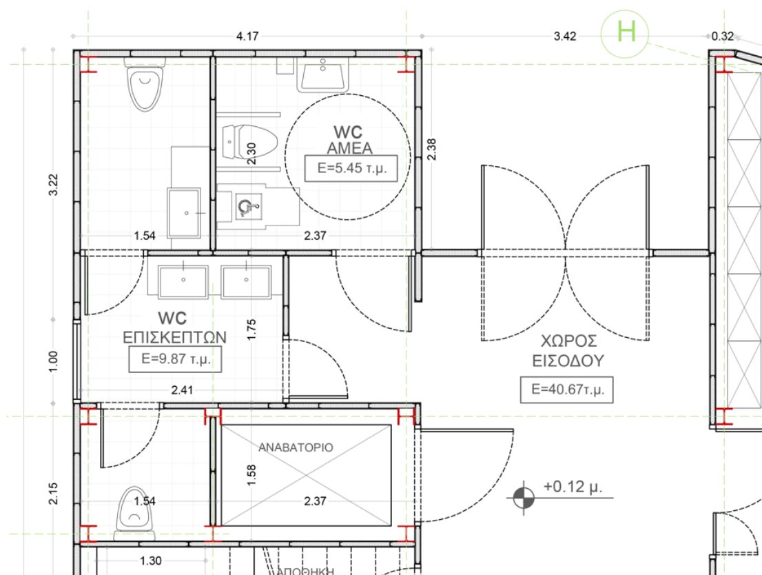
Εικόνα 5: Χώροι ισογείου (WC) στους οποίους θα πραγματοποιηθεί επικάλυψη με πλακίδια.
