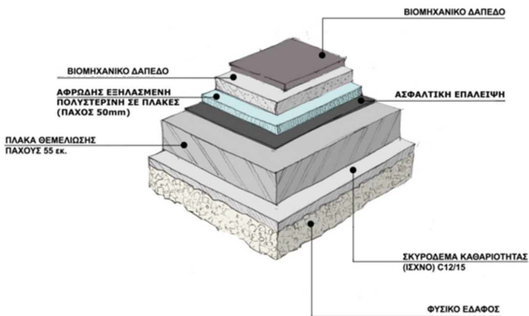
Εικόνα 4: Λεπτομέρεια δαπέδου στο ισόγειο σύμφωνα με την αρχιτεκτονική μελέτη.
